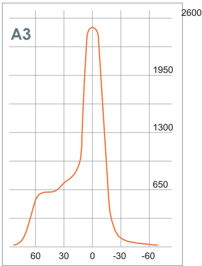
Křivky svítivosti
